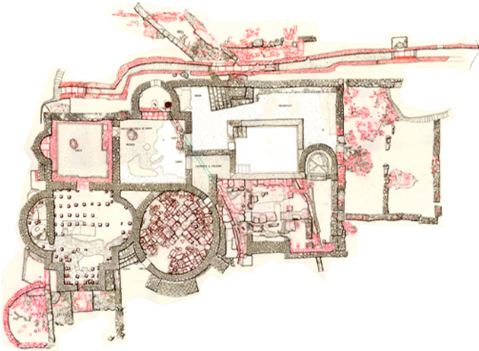
Nova Siri. Impianto termale di Ciglio dei Vagni. Pianta generale
